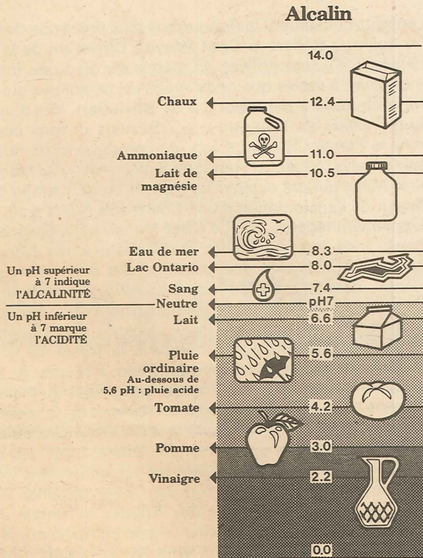
L'échelle pH (de 0 à 14) sert à mesurer les ions hydrogènes libres dans une solution
