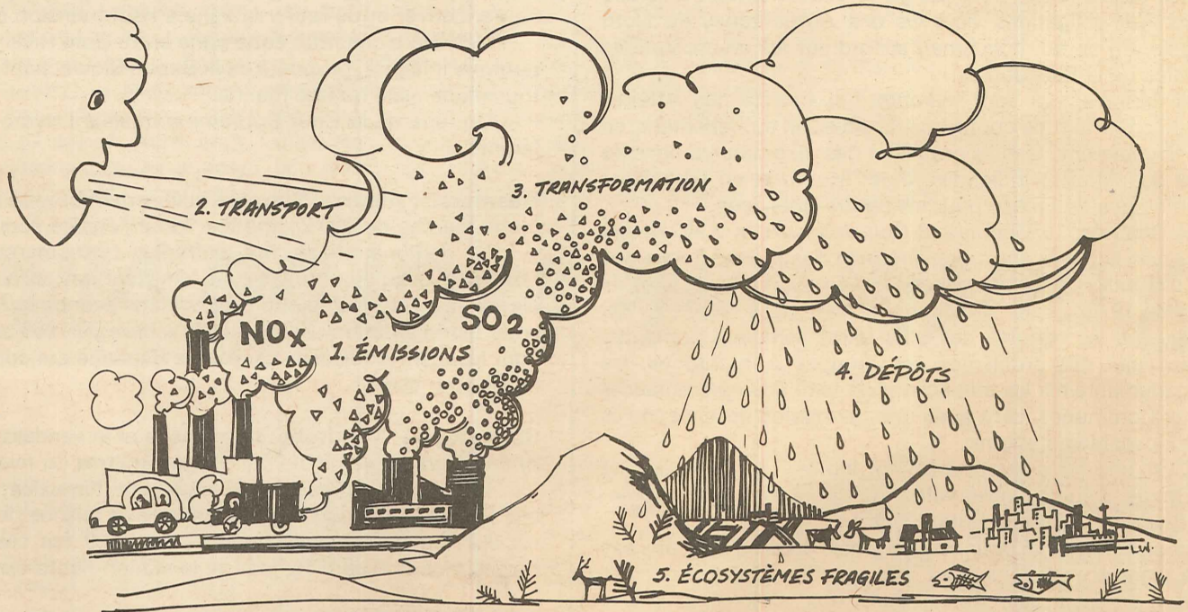
LES VENTS TRANSPORTENT LES POLLUANTS SUR DES DISTANCES... DE PLUSIEURS CENTAINES ET MÊME PLUSIEURS MILLIERS DE KILOMÈTRES
